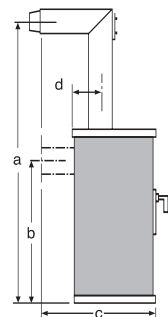
Maß a und c: mit Original-Winkelrohr dimension a and c: with original angle pipe Côtés a et c : avec conduit coude d'origine Wymiary a i c : z oryginalną rurą pod kątem 90°
